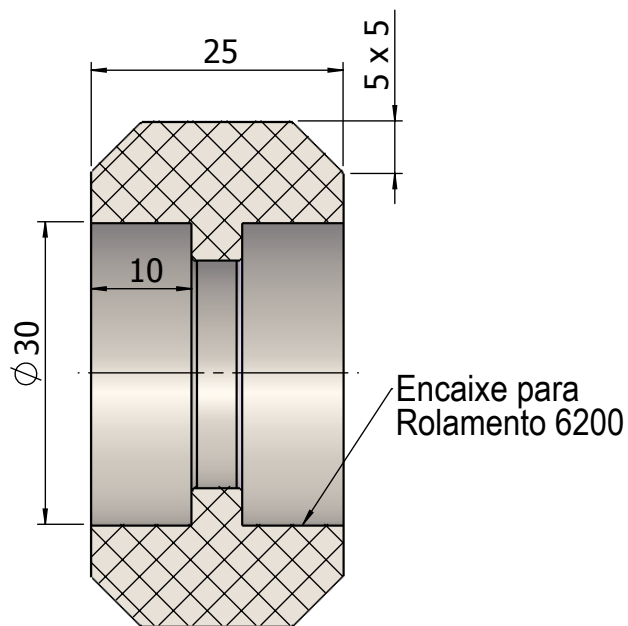
SEÇÃO A-A
